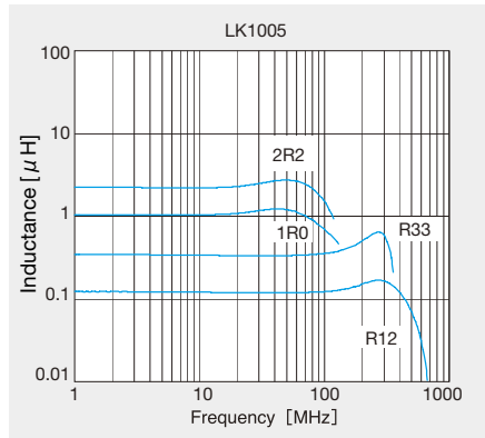
インダクタンス周波数特性例 Inductance-vs-Frequency characteristics (Measured by HP4294A or HP4291A)
