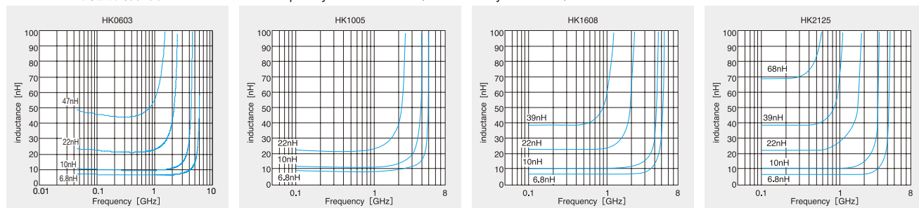
インダクタンス周波数特性例 Inductance-vs-Frequency characteristics (Measured by HP8719C)
